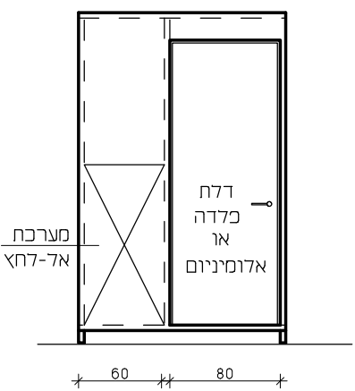
חזית C
