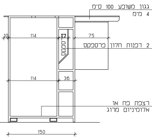
חזית E
