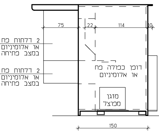
חזית B
