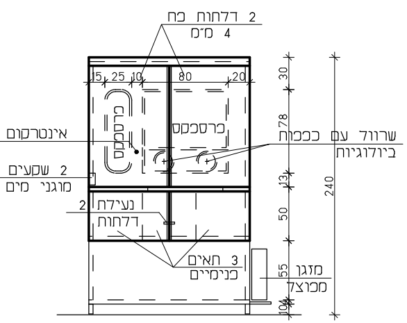
חזית A
