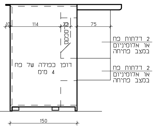
חזית D
