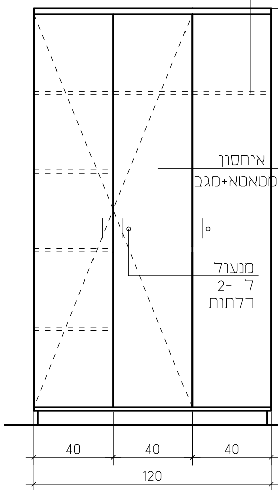
חזית ק.מ. 1:20
