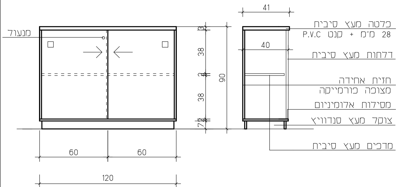
חזית ק.מ. 1:20
