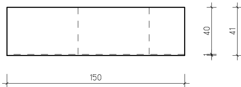
תבנית ק.מ. 1:20
