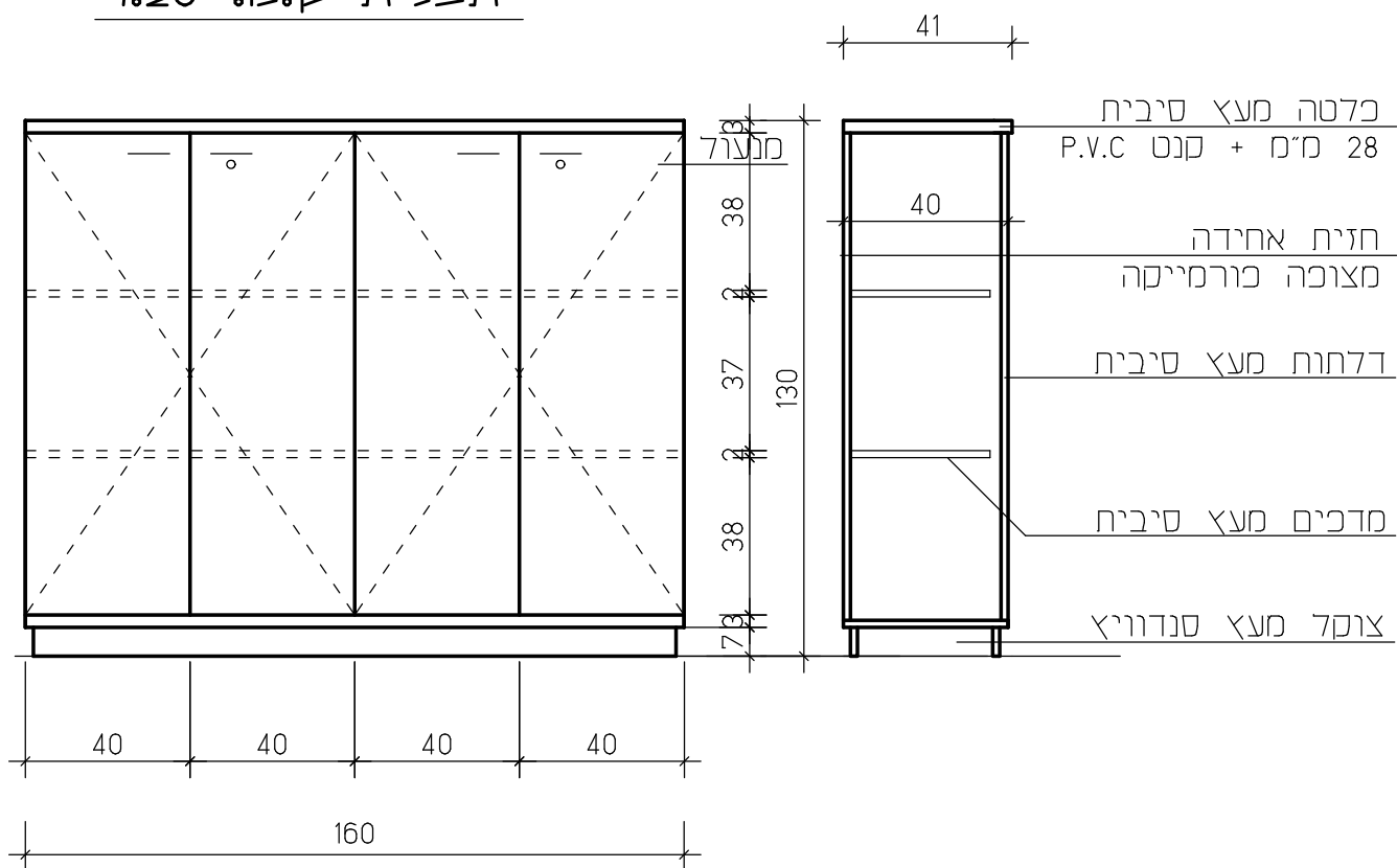
תבנית ק.ב. 1:20
