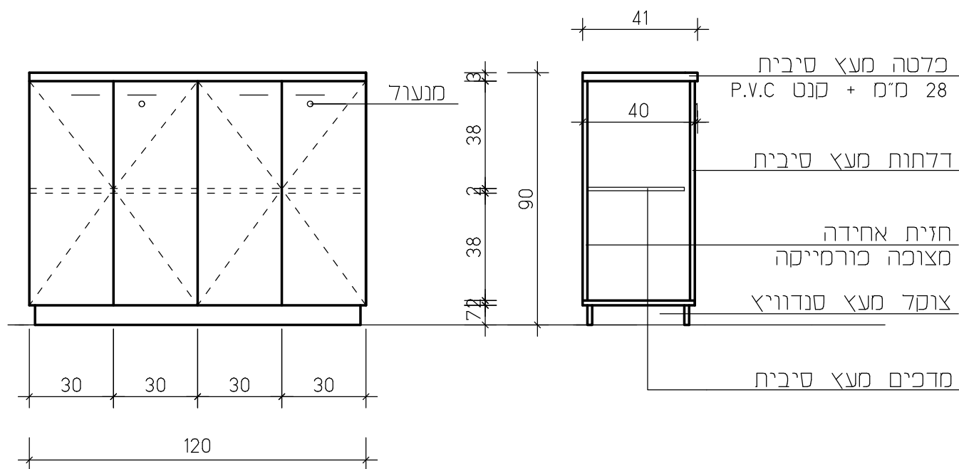
חזית ק.מ. 1:20
