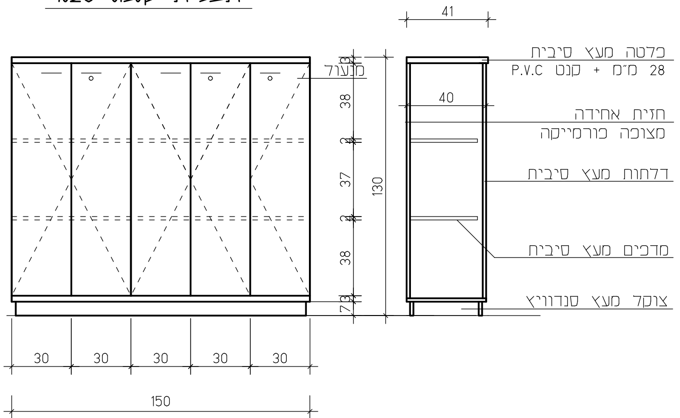
תבנית ק.מ. 1:20
