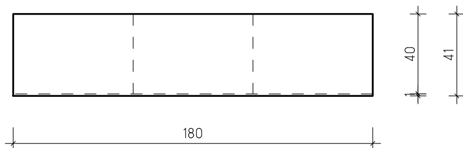
תבנית ק.ב. 1:20
