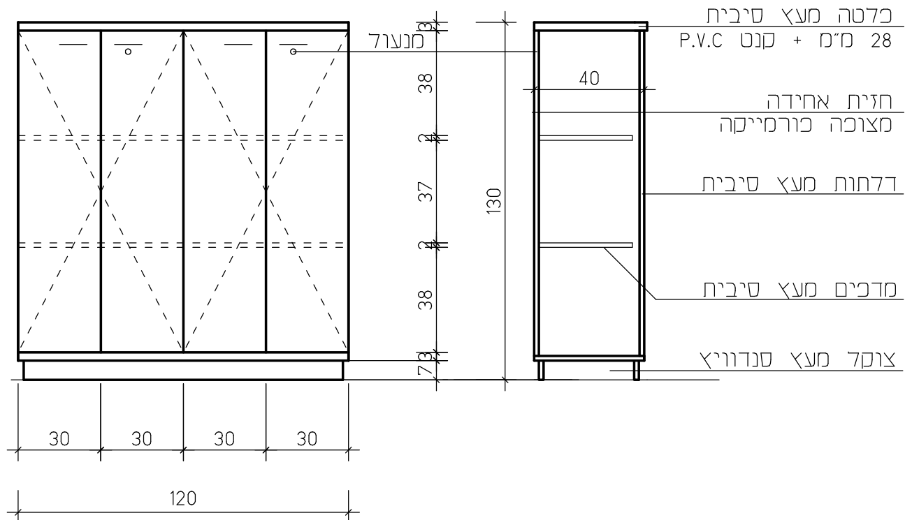
תבנית ק.מ. 1:20
