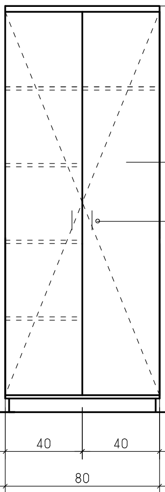
חזית ק.מ. 1:20
