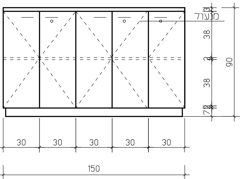
חזית ק.ב. 1:20
