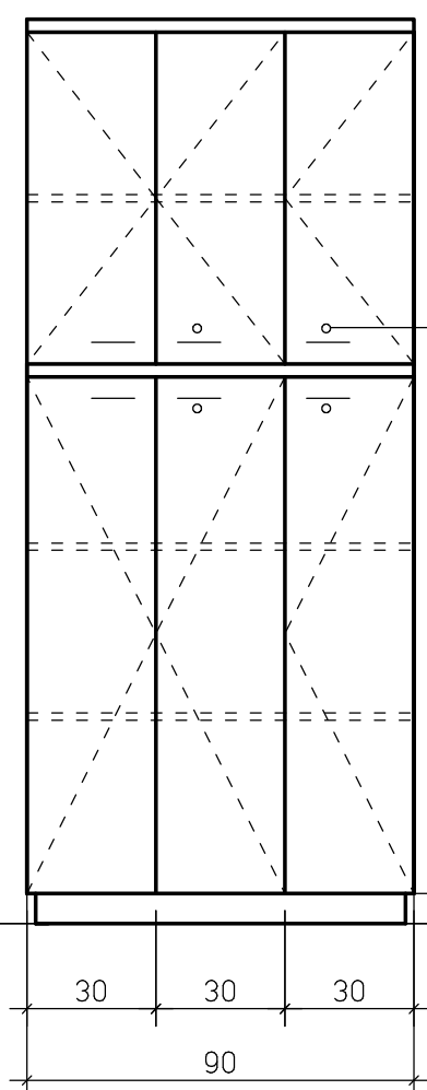
תבנית ק.מ. 1:20
