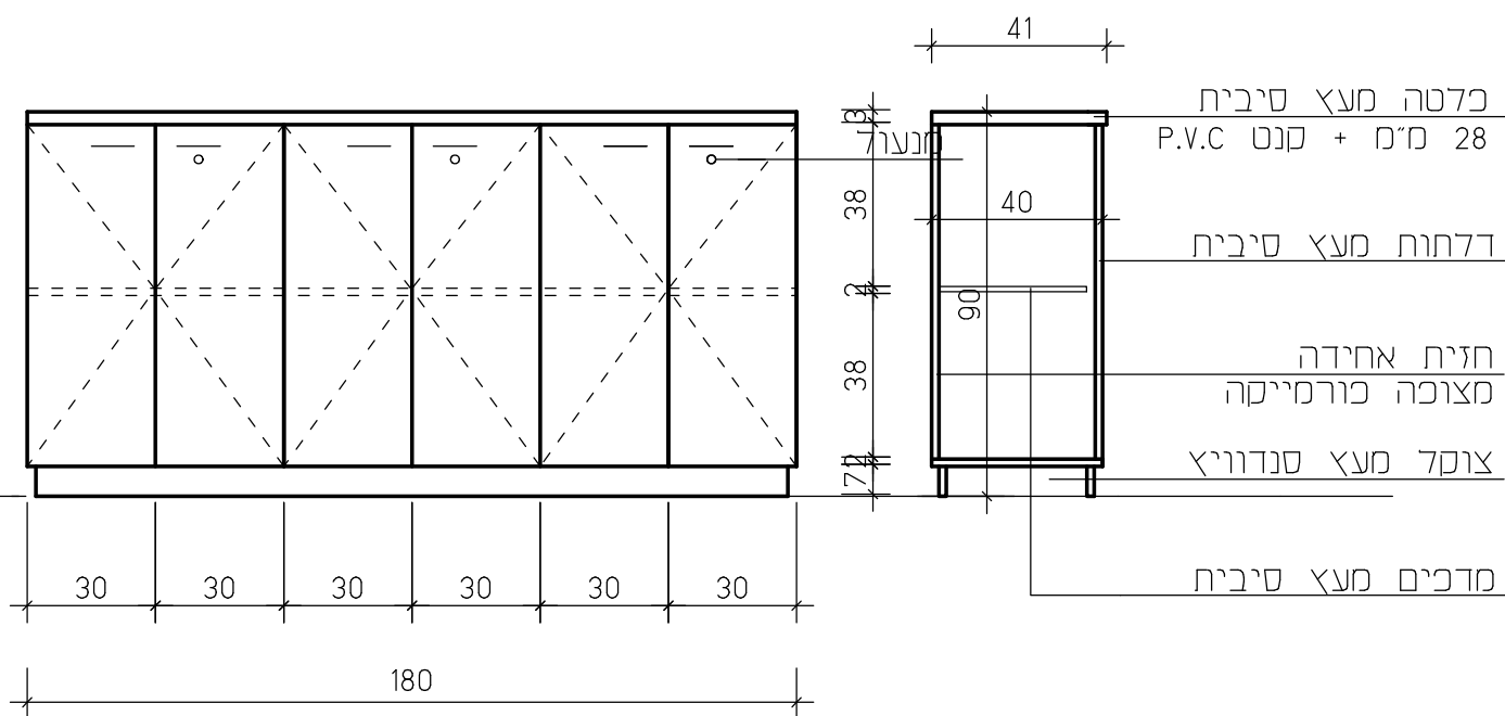
חזית ק.מ. 1:20
